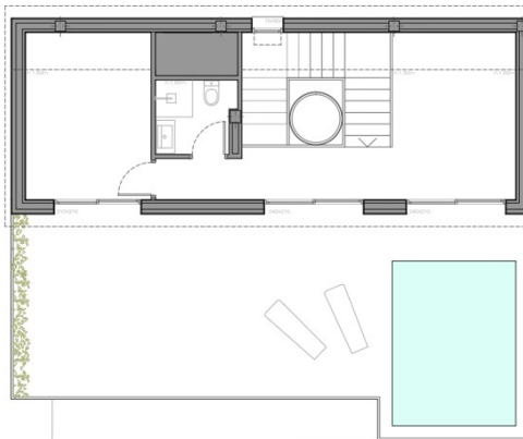
PLANTA GOLFA
