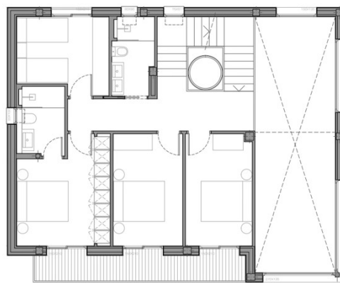
PLANTA PRIMERA
