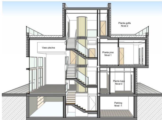
Seccion
