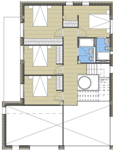
Planta primera
